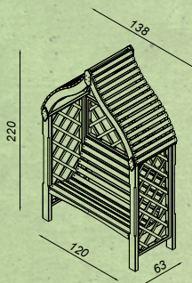
Siam Arbour 40190
