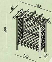
Linton Arbour 40182
