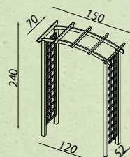
Olimpia Arch 41100
