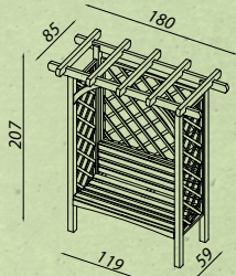
York Arbour 40181
